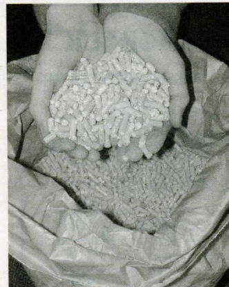
Holzpellets – der Brennstoff der Zukunft. Für die Holzpresslinge legt eine eigene Norm DIN 51731 die Qualität fest. Sie garantiert, dass der Brennstoff wirklich nur aus Sägespänen ist.
